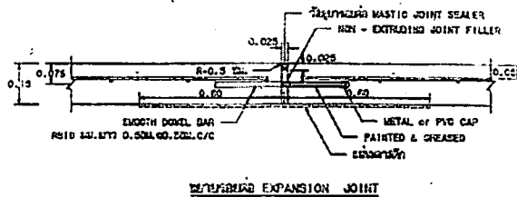
ขยายแสดง EXPANSION JOINT
