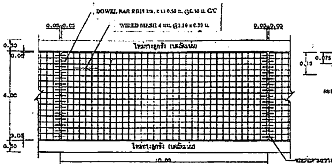
รูปเขียนแสดงการเสริมเหล็กและโครงข่าย
